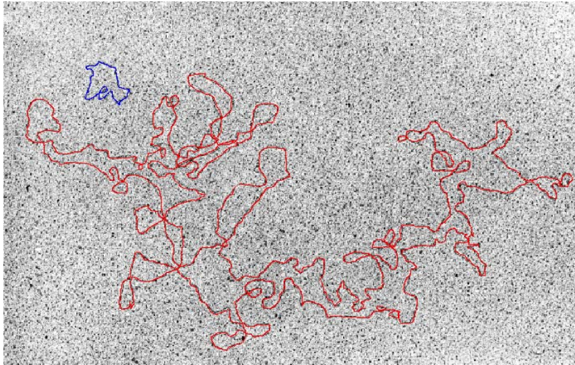
EM of Arthrobacter nicotivorans plasmid pAO1
